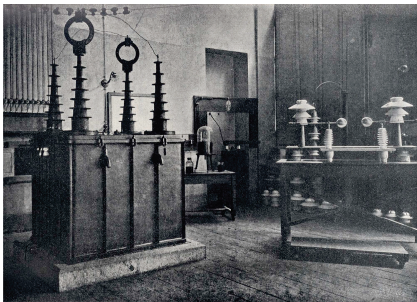
Laboratorio di Elettrotecnica sviluppato sulla prima Scuola fondata da Galileo Ferraris al Castello del Valentino, ASPoliTO, Archivio Storico Politecnico di Torino.
