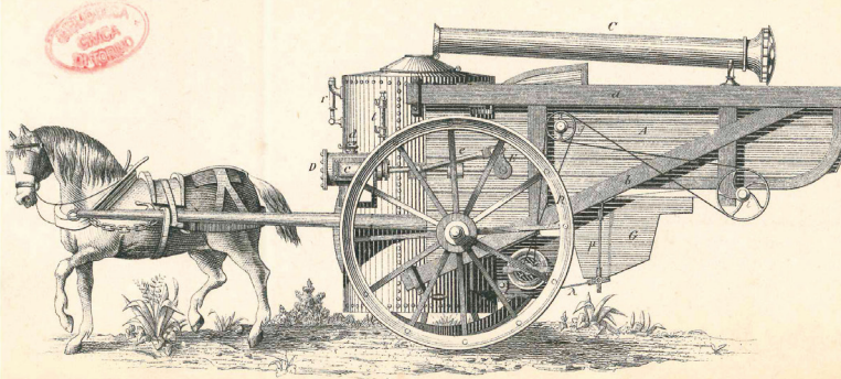
Fig. 1. Elevazione longitudinale (dalla parte ove trovasi il cilindro motore.)
