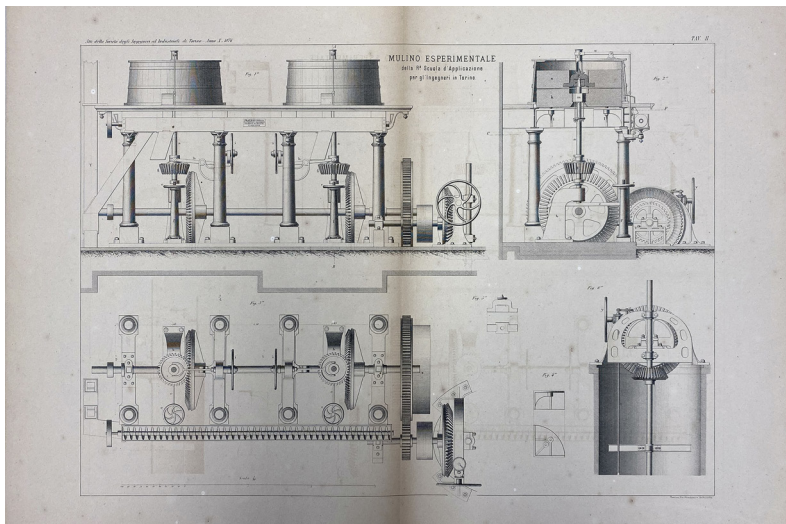
Giovanni Curioni, docente di Costruzioni civili, idrauliche e stradali, progetta il mulino sperimentale per lo studio dei macinati e delle relative tasse per il nuovo Regno d'Italia. G. Curioni, Molino sperimentale nella R. Scuola d'applicazione degli Ingegneri in Torino , in "Atti della Società degli ingegneri e degli industriali di Torino", 1876, pp. 51-61.
