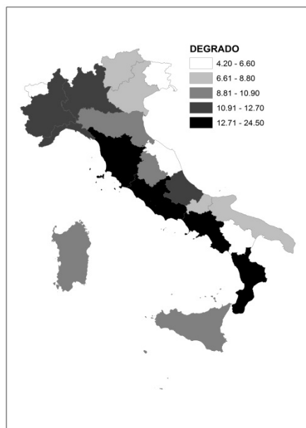
Figura 1C - Mappe indicatori 9-11
